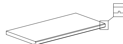
GRADONE BORDO COSTA CON SGOCCIOLATOIO 50x100 cm - 20"x39" GRIP RETT. ● 202
