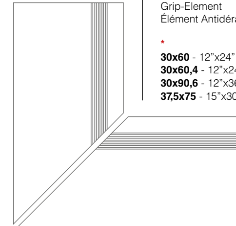
Bordo Becco Fully rounded edge Runde Kante Bord Rond
