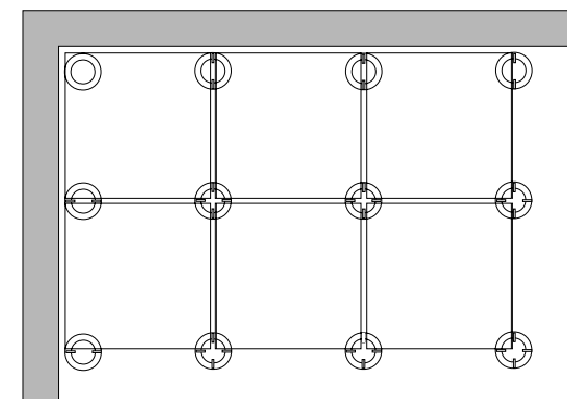
SUPPORTO REGOLABILE AUTOLIVELLANTE Paving support Verstellbare Stütze Support réglable Soporte regulable Регулируемая опора
